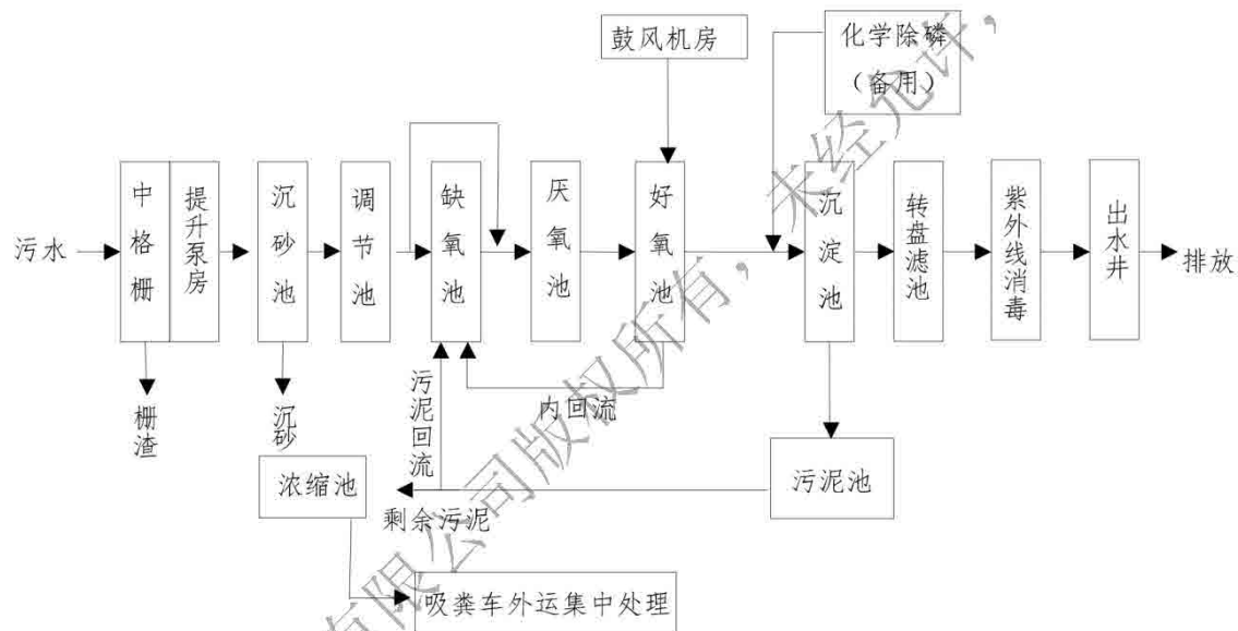
图 8 污水处理工艺流程图
