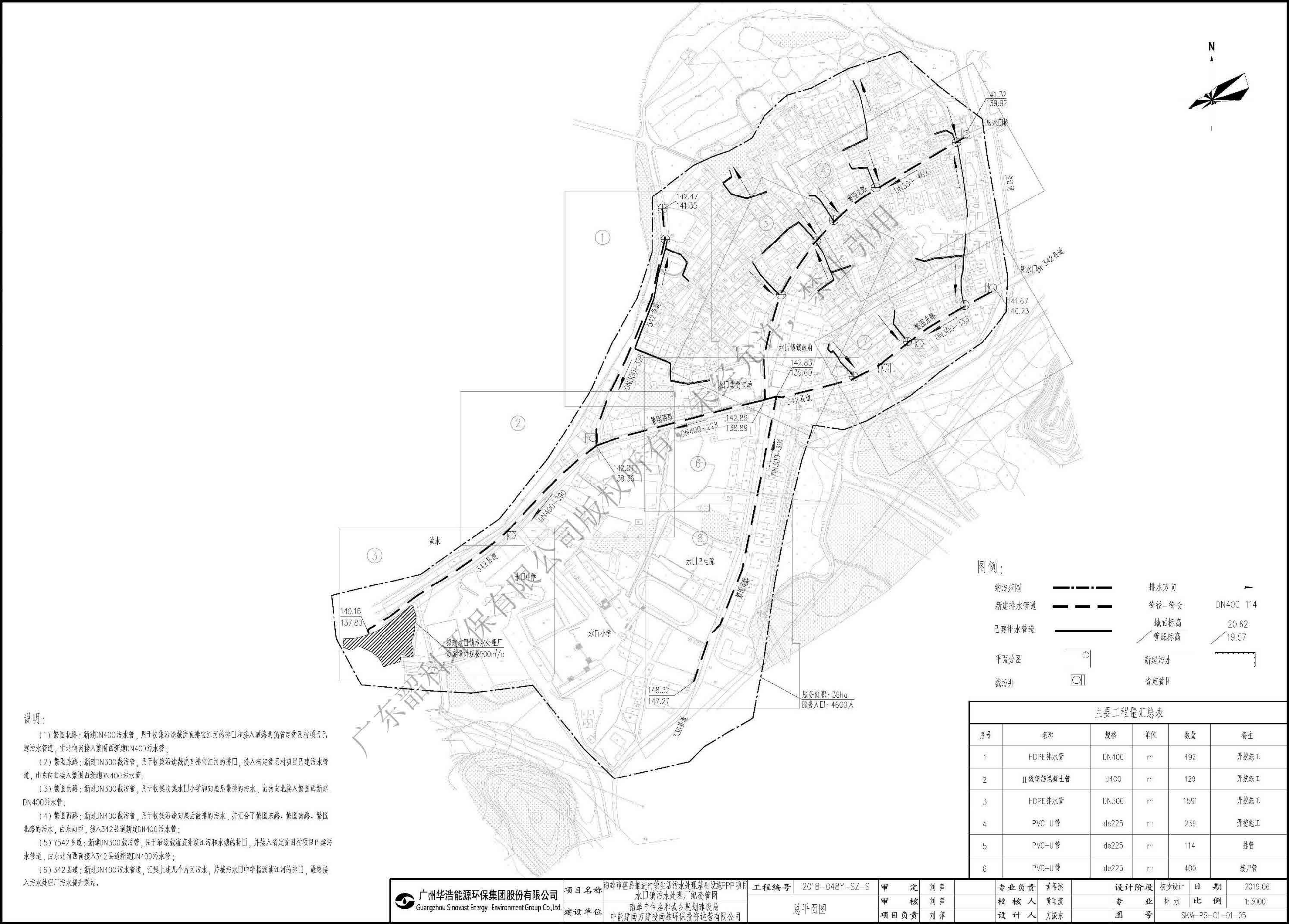
图 3 水口镇污水处理厂配套管网示意图
